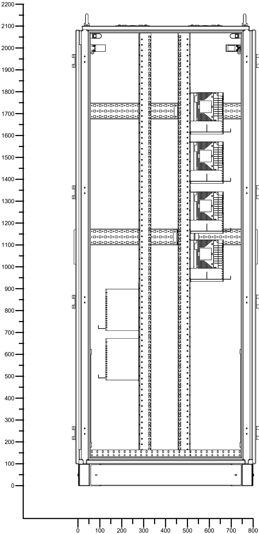
Вид справа
