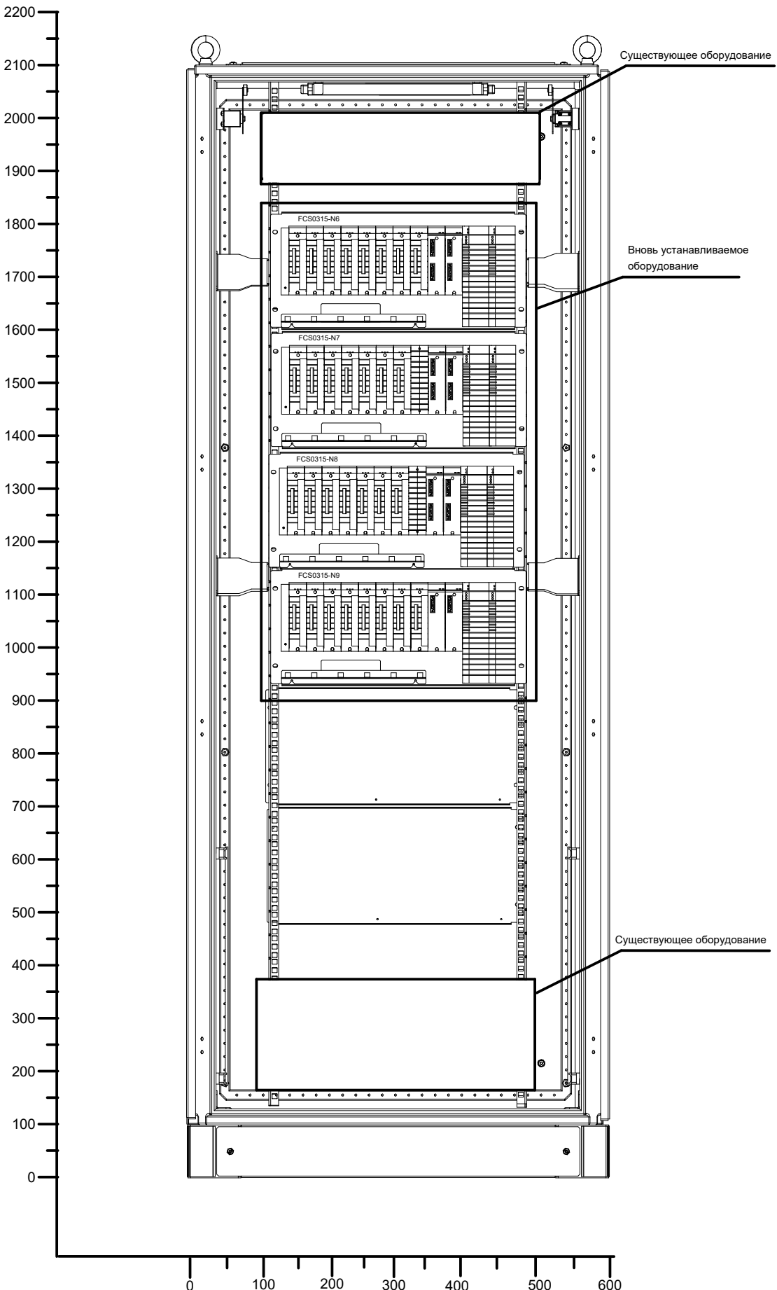
Вид сзади без дверей
