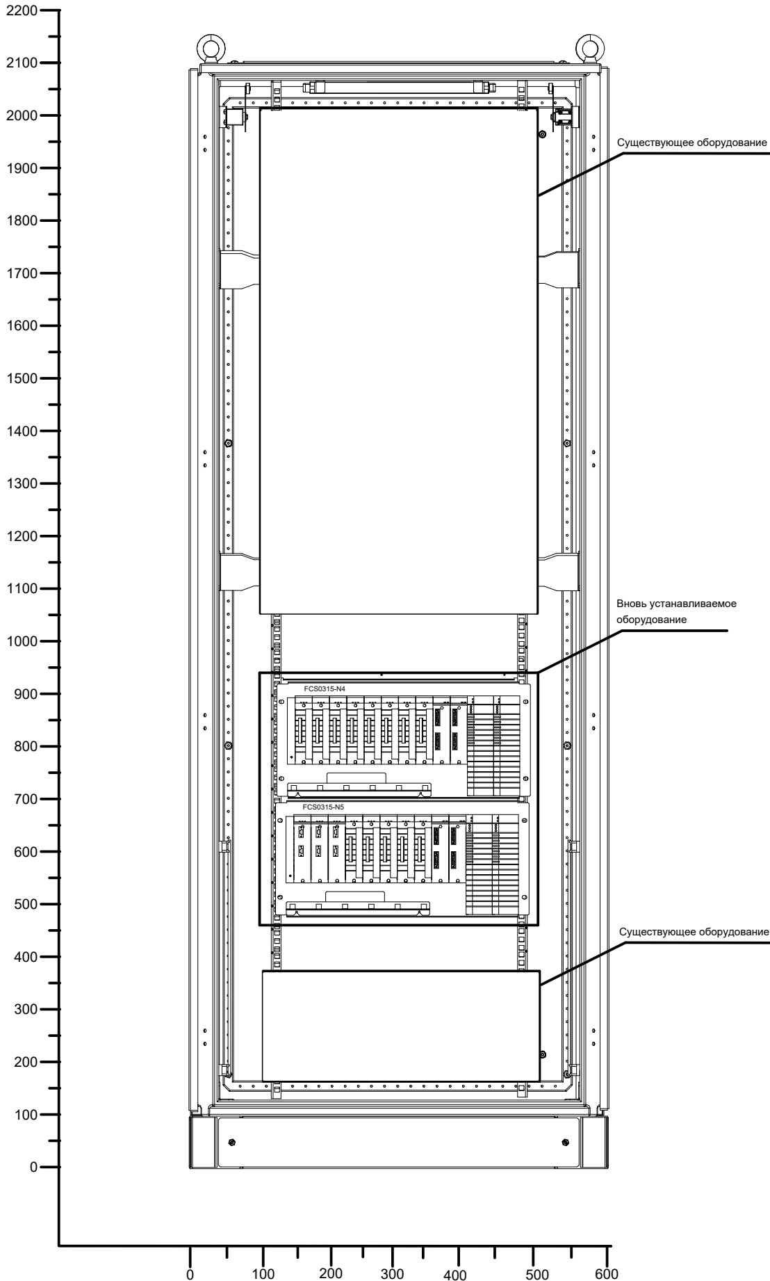
Вид спереди без дверей
