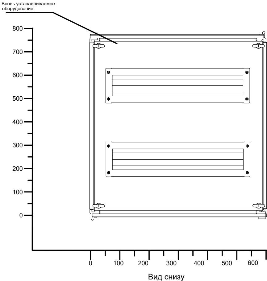
Вид снизу
